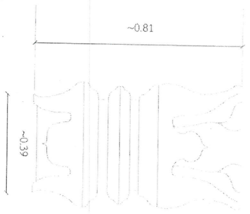
แบบขยายบัวหัวเสา NO SCALE
